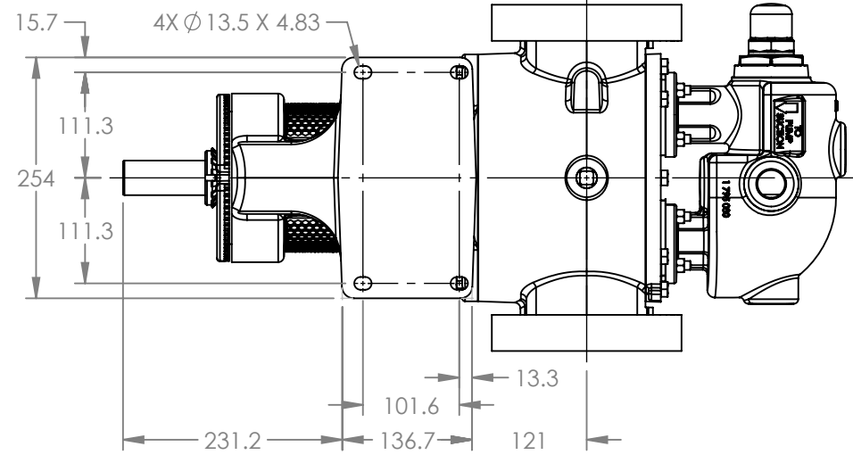
VIEW A-A
