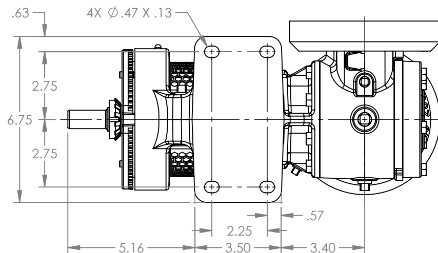
VIEW A-A
