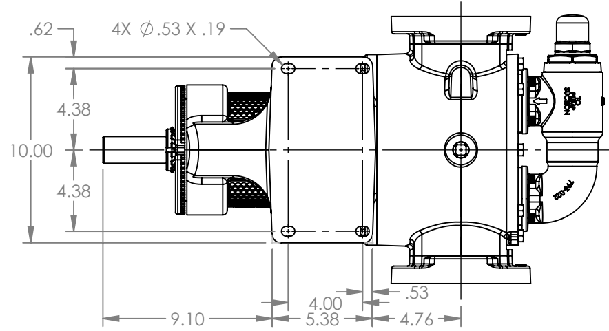
VIEW A-A
