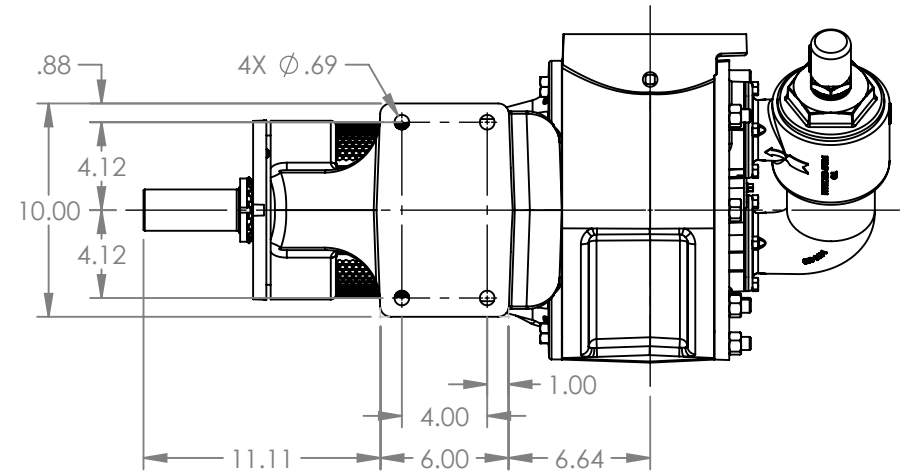
VIEW A-A
