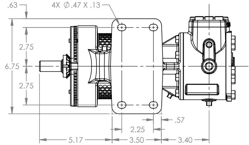
VIEW A-A
