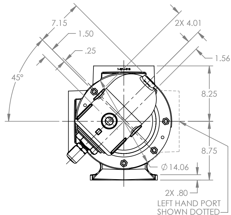
VIEW A-A
