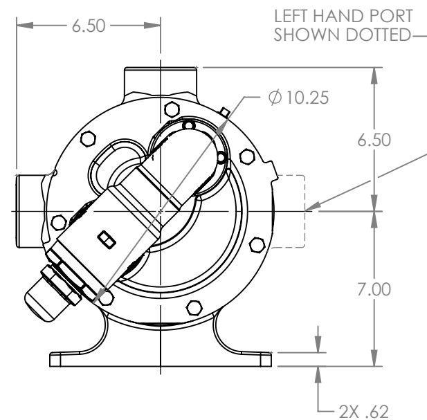
VIEW A-A
