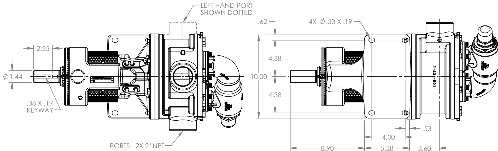
VIEW A-A
