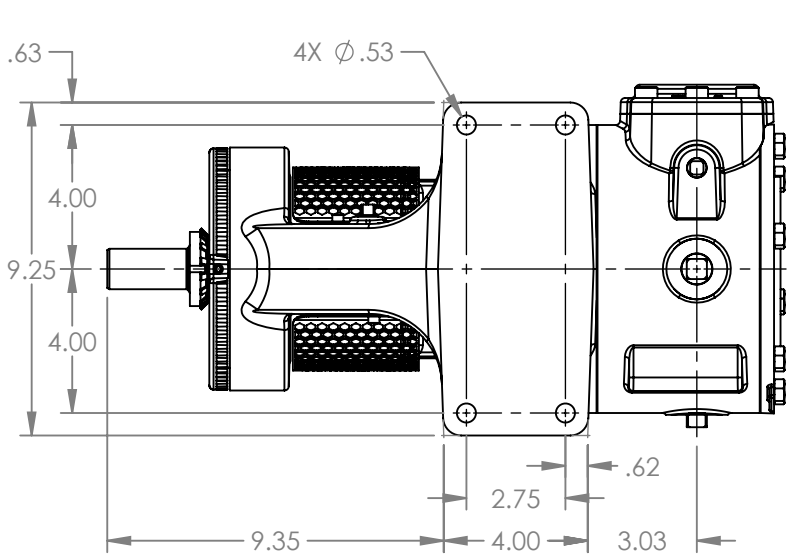
VIEW A-A
