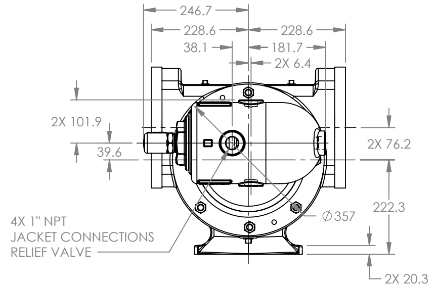
VIEW A-A
