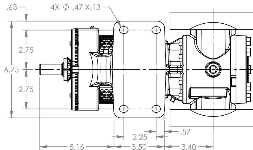
VIEW A-A
