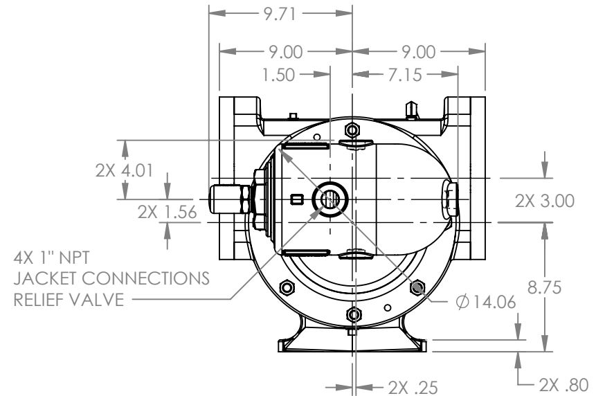
VIEW A-A
