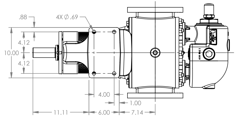
VIEW A-A
