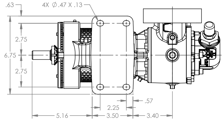
VIEW A-A
