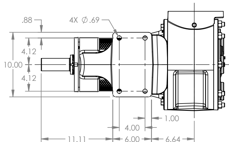
VIEW A-A
