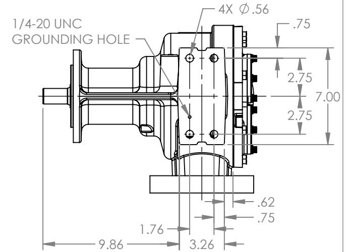
VIEW A-A
