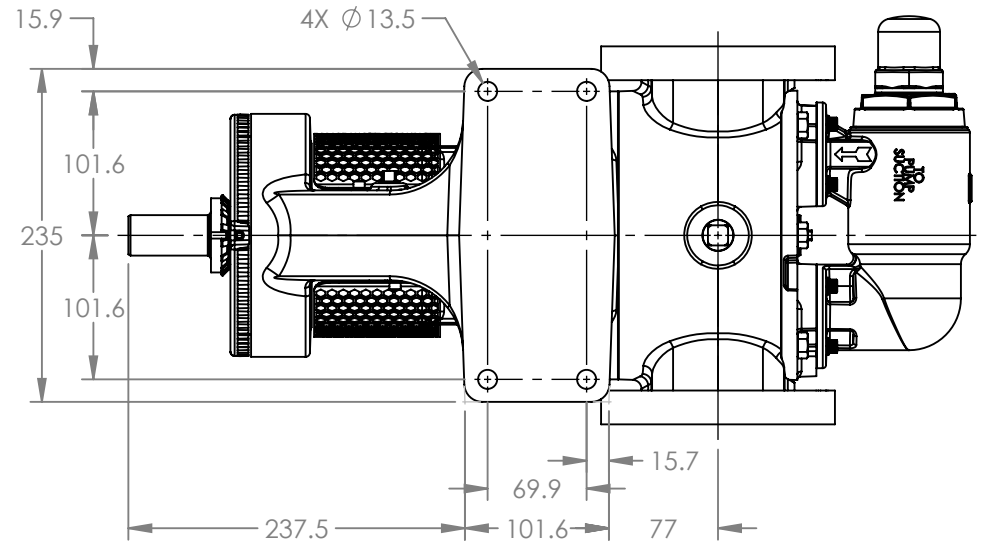
VIEW A-A
