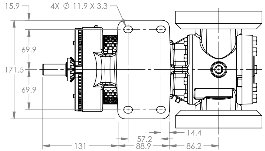
VIEW A-A
