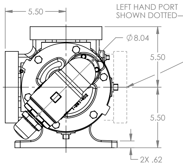
VIEW A-A
