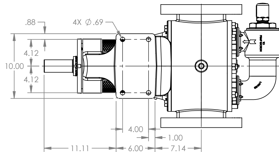
VIEW A-A
