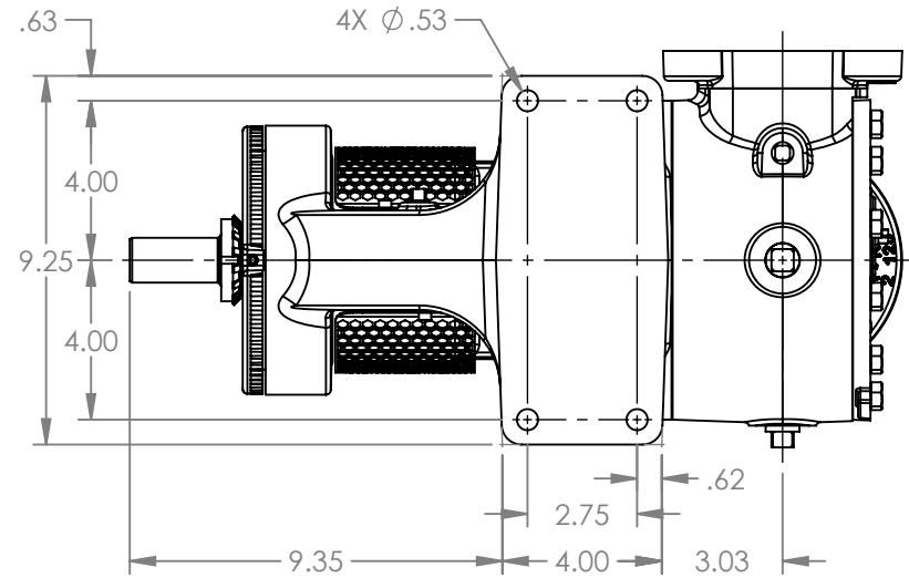
VIEW A-A
