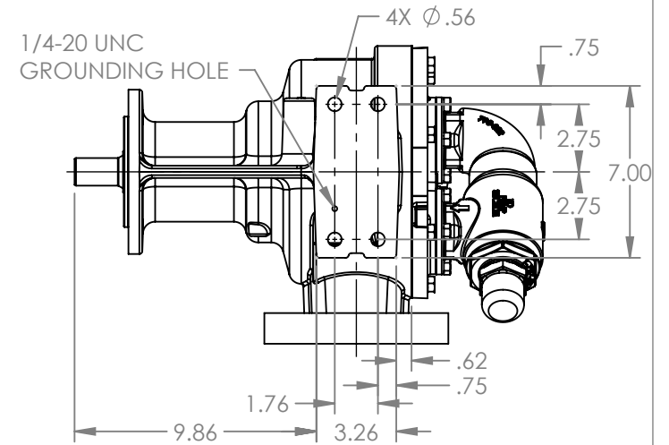
VIEW A-A
