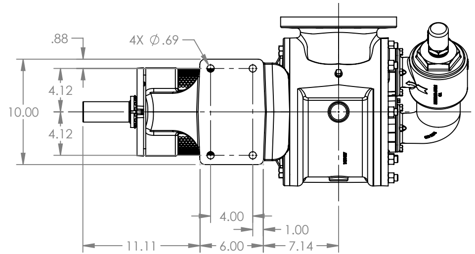
VIEW A-A
