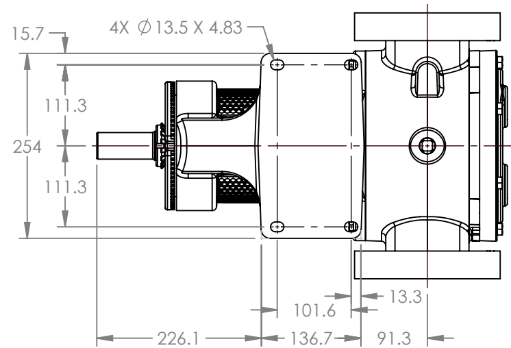
VIEW A-A
