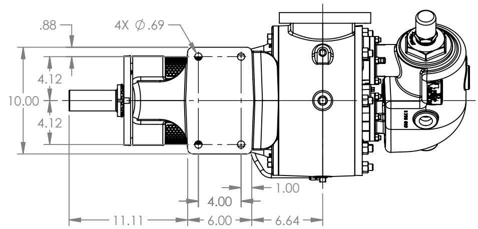
VIEW A-A
