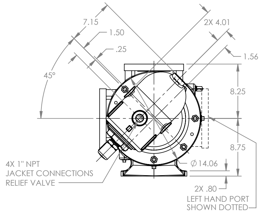
VIEW A-A
