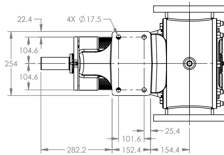
VIEW A-A
