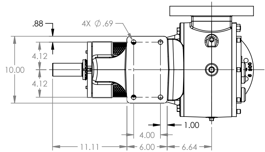
VIEW A-A
