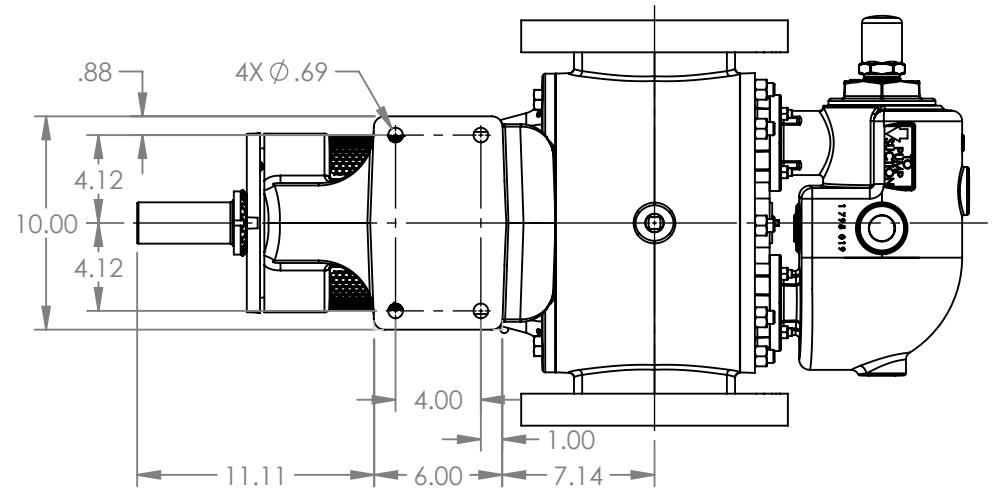
VIEW A-A
