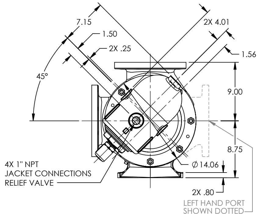
VIEW A-A
