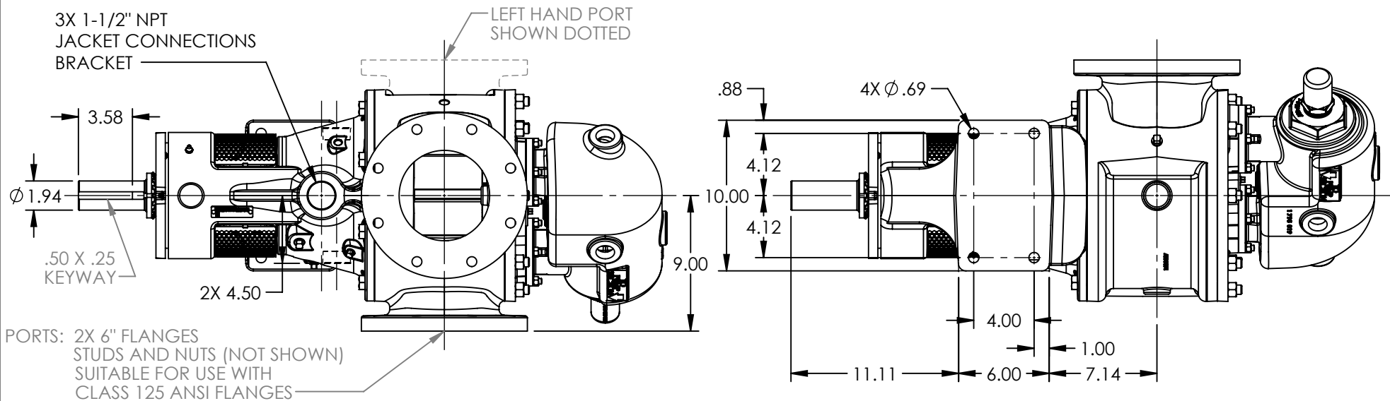
VIEW A-A
