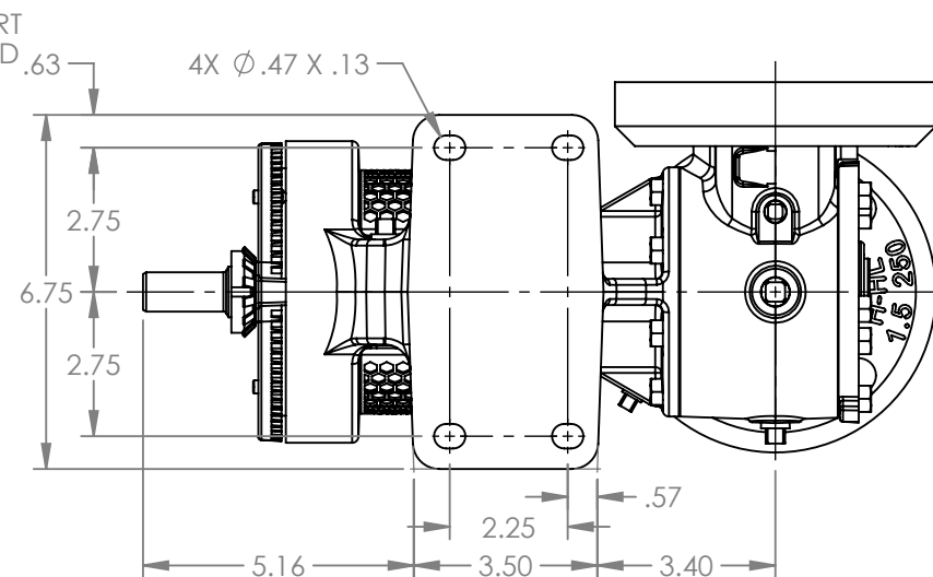
VIEW A-A
