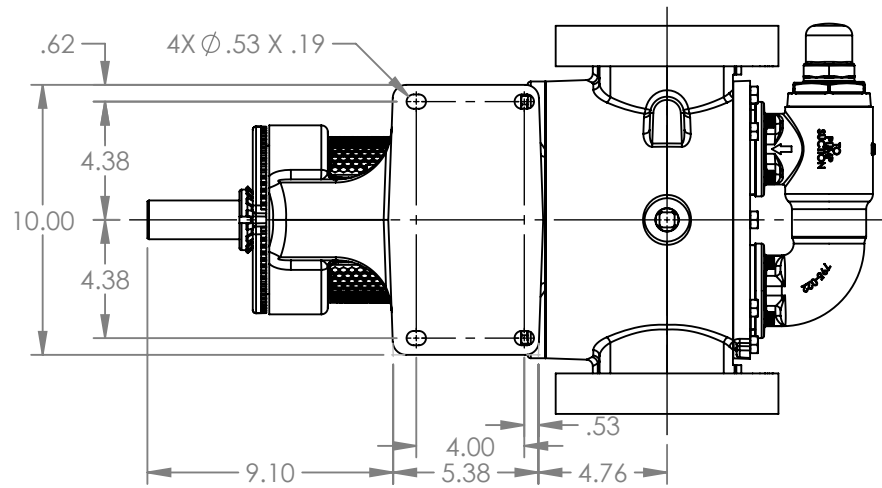
VIEW A-A
