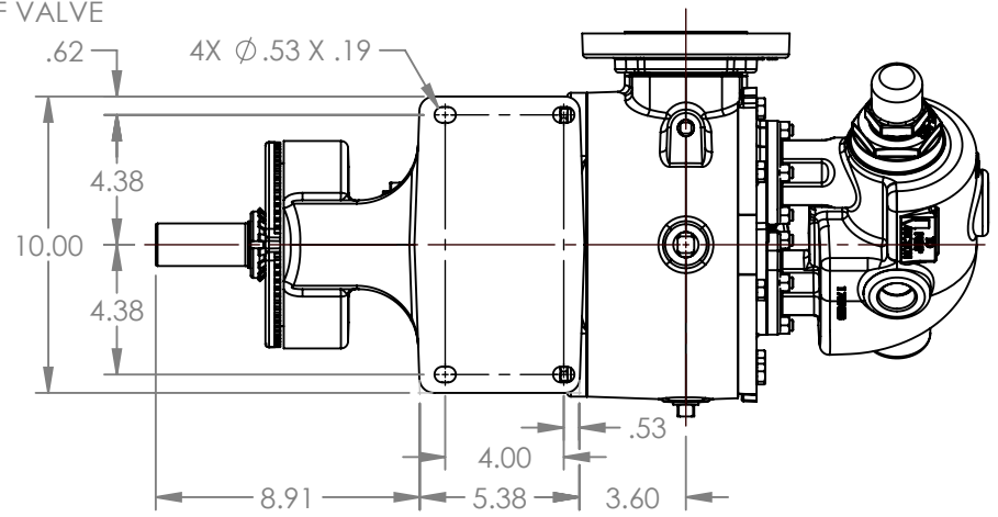
VIEW A-A
