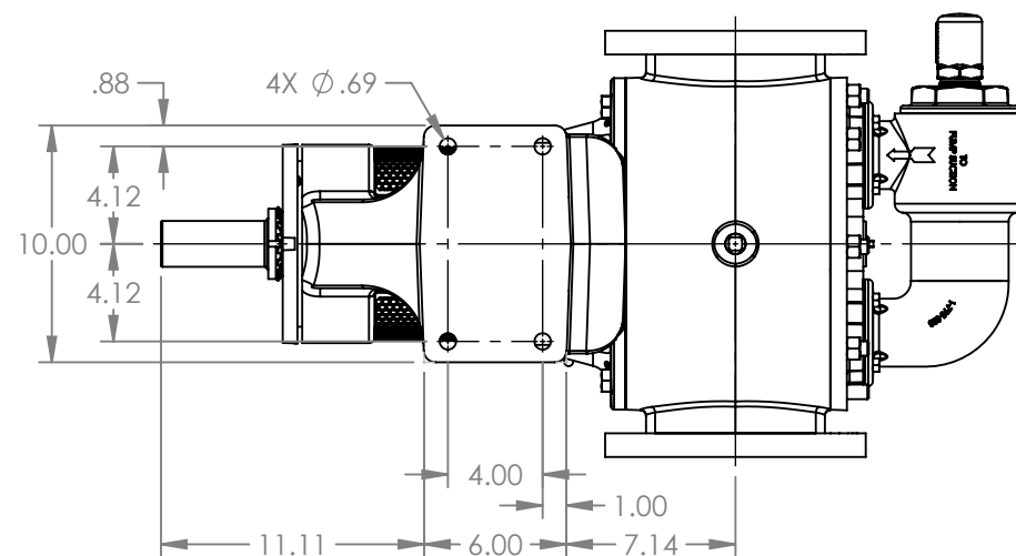
VIEW A-A
