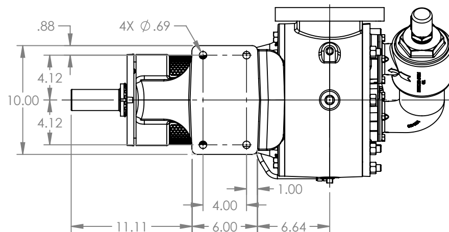
VIEW A-A
