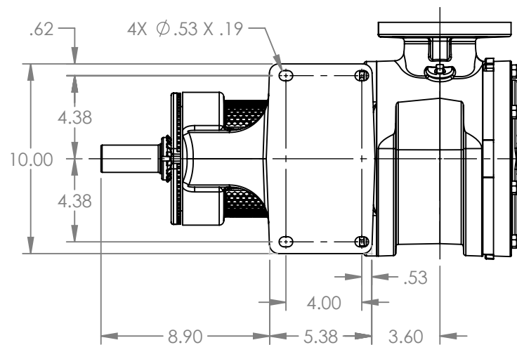
VIEW A-A
