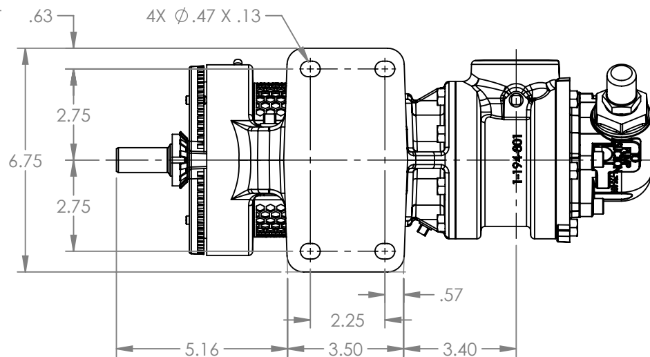
VIEW A-A
