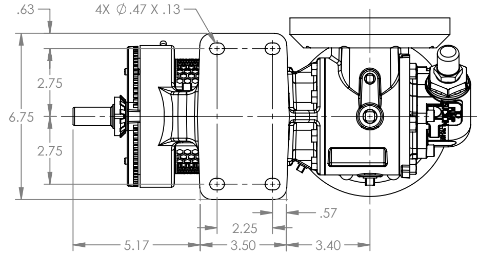
VIEW A-A
