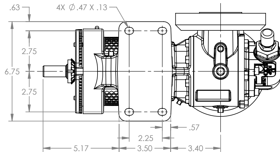
VIEW A-A
