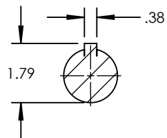
SECTION A-A SCALE 1 : 4
