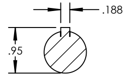
SECTION A-A SCALE 1 : 2
