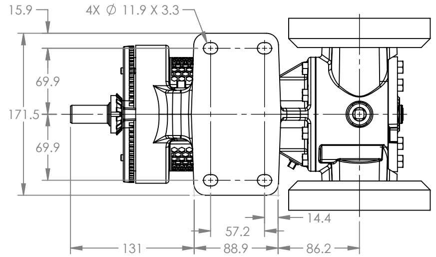
VIEW A-A
