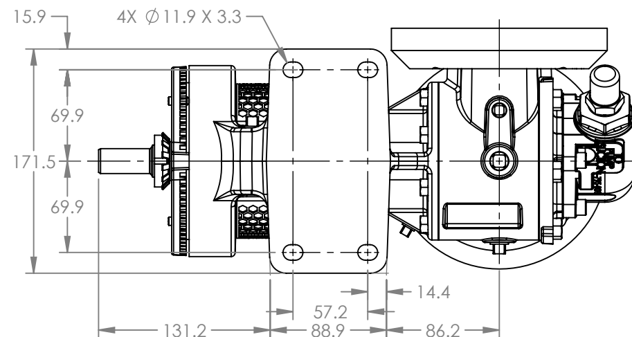
VIEW A-A
