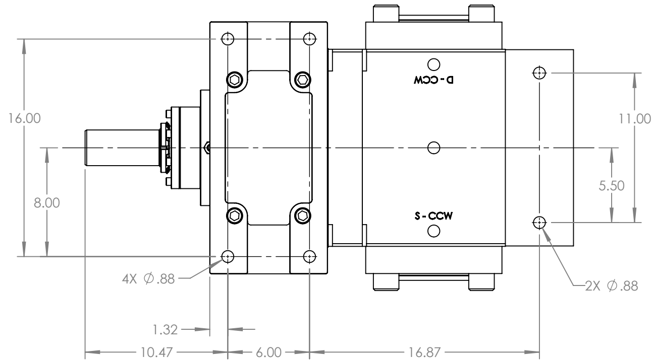
VIEW A-A
