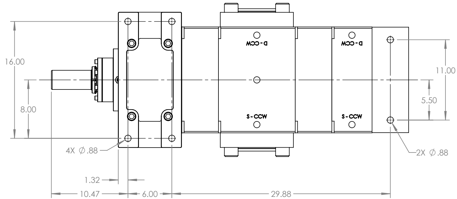
VIEW A-A
