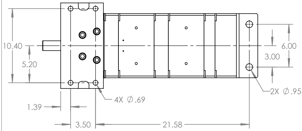
VIEW A-A
