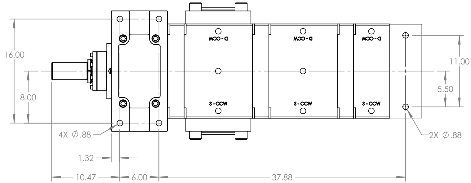
VIEW A-A
