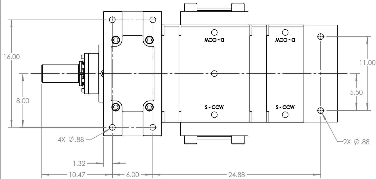
VIEW A-A
