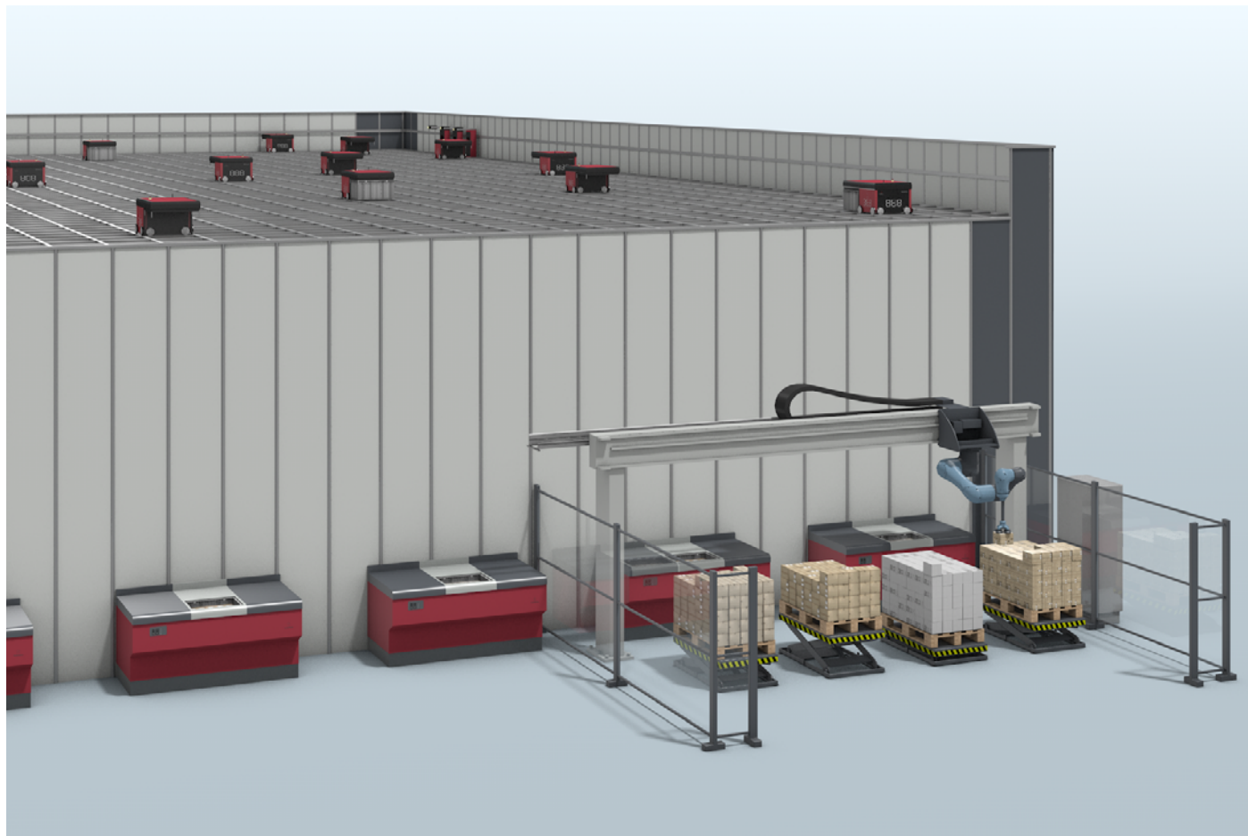
Automatizované řešení s robotickým systémem pro vyzvednutí a umístění za účelem (de-)paletizace
