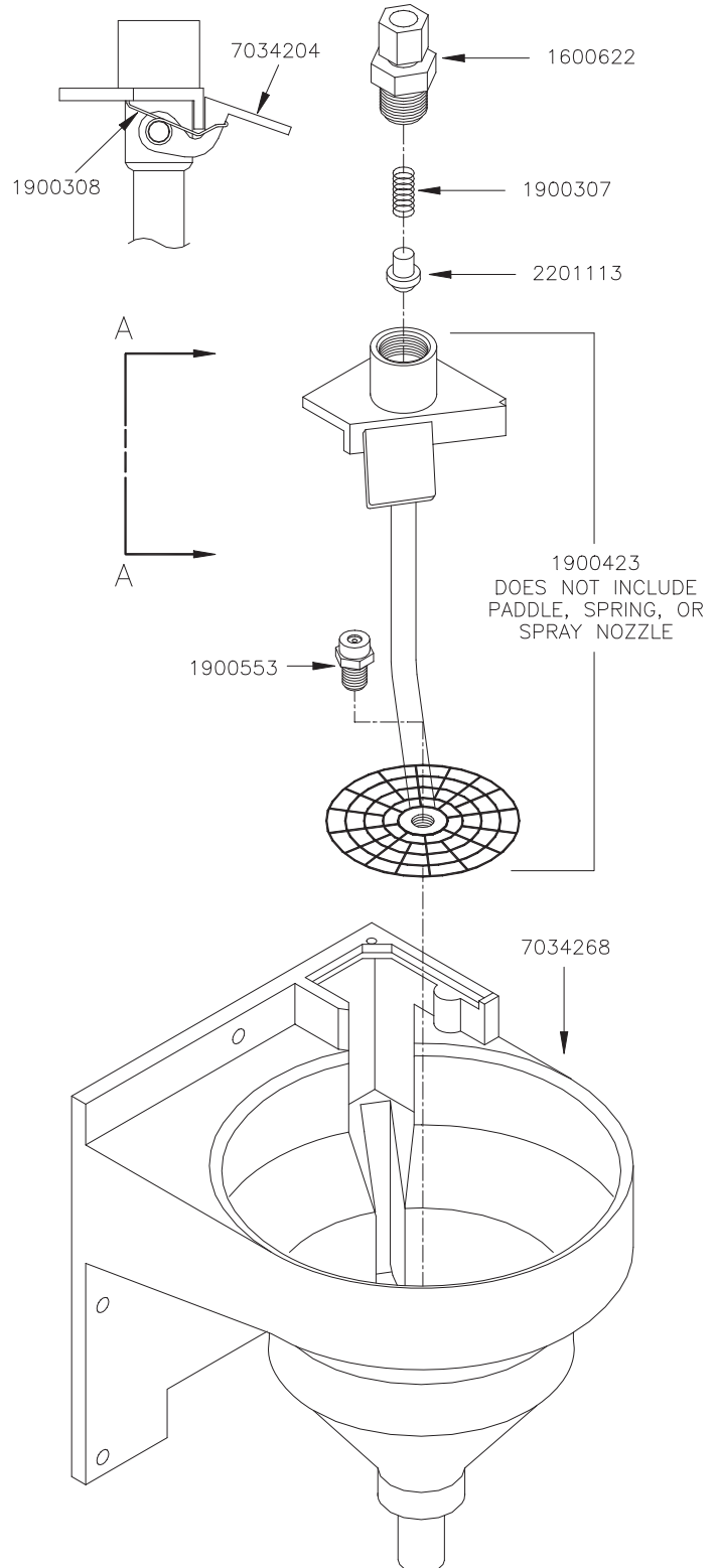
VIEW A-A
