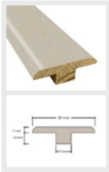
T-Mold
