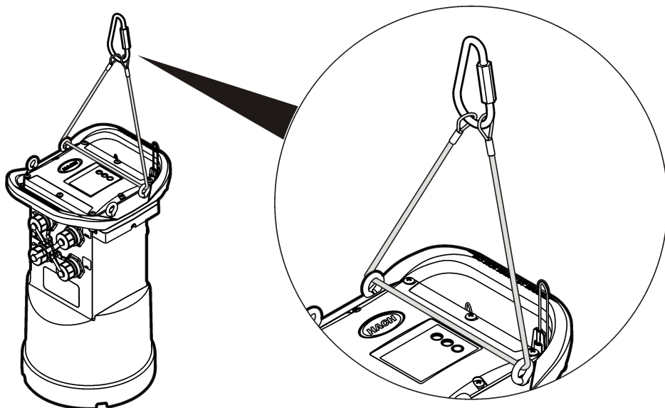
Slika 13 Obesite zapisovalnik s kabla.
