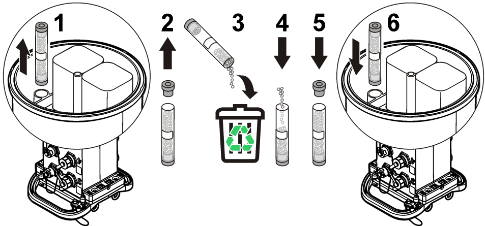
Figura 14 Sostituzione dell'essiccante
