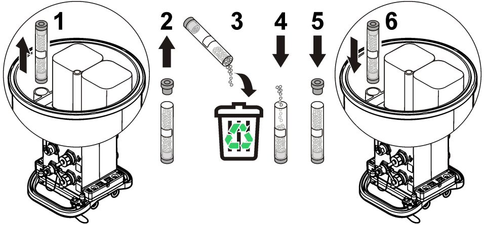
Şekil 14 Kurutucunun deęiřtirilmesi
