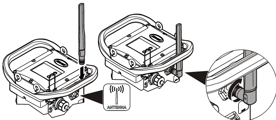
Slika 10 Namestitev antenskega lista
