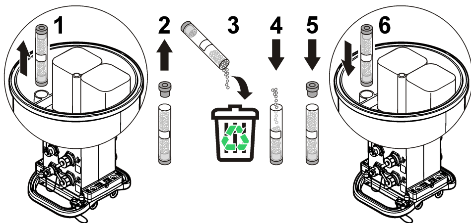
Slika 14 Zamenjava sušila
