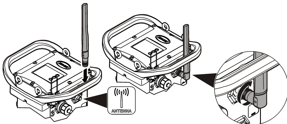
Slika 10 Priključite plosnatu antenu (blade)
