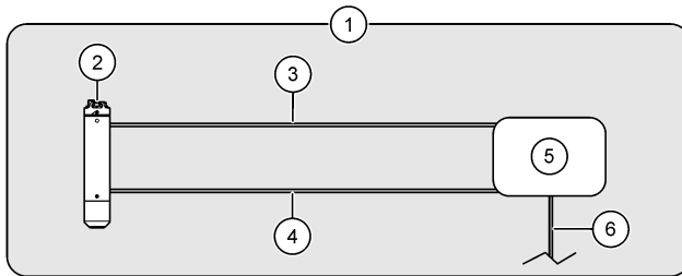
Abbildung 5 Feldtransmitter Cx440EX
