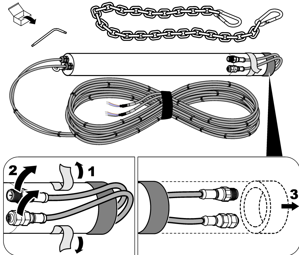
Figur 4 Anslut kabelskyddet
