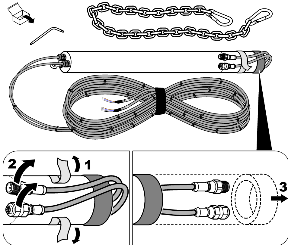
Obr. 4 Připevňte chránič kabelu
