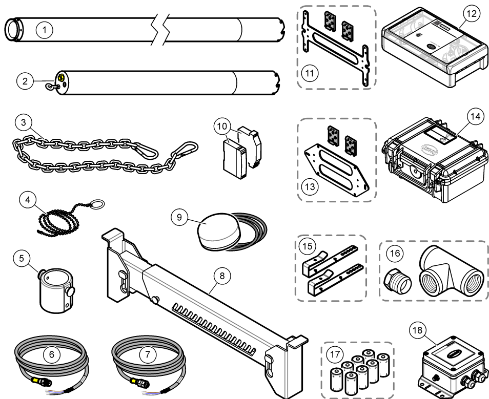
Εικόνα 3 Παρελκόμενα
