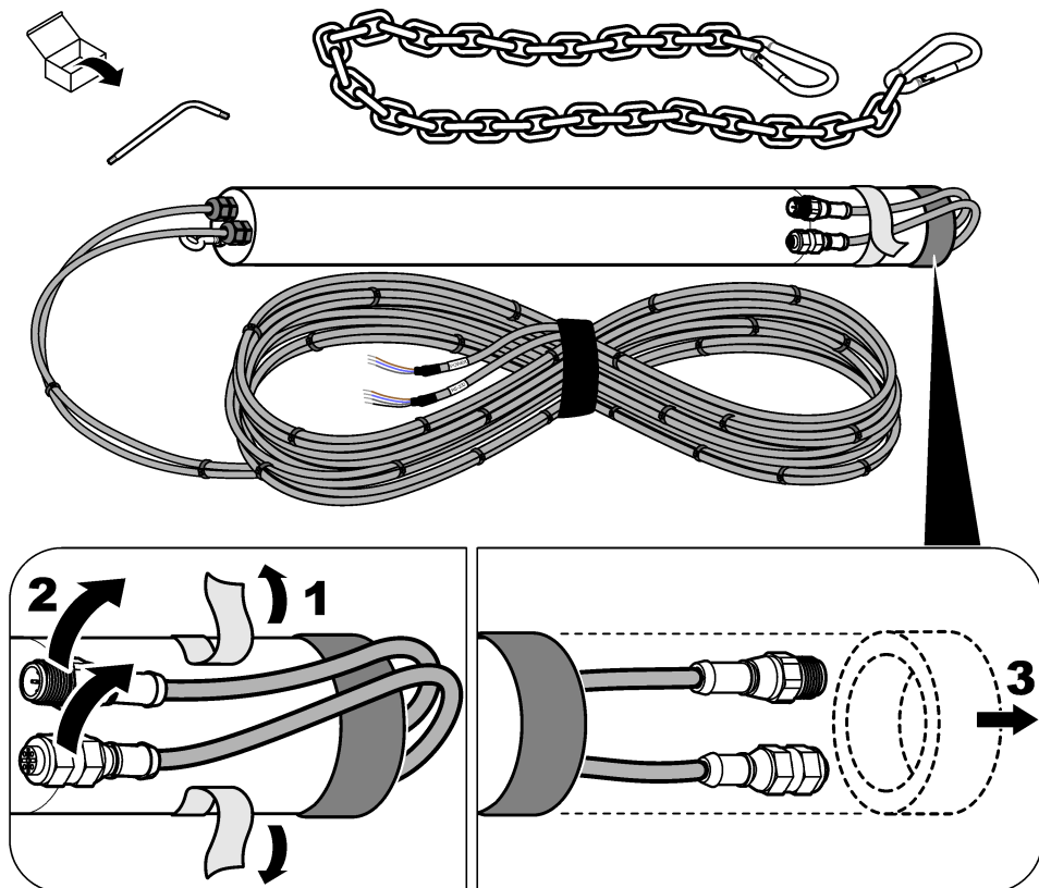
Obrázok 4 Upevnenie krytu kábla
