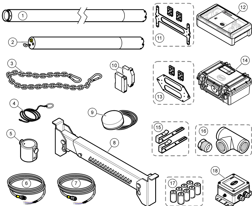
Figur 3 Tilbehør
