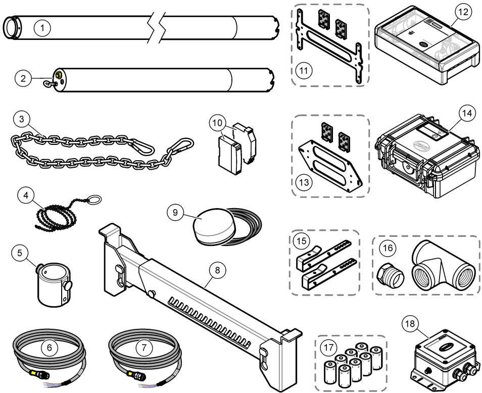
Abbildung 3 Zubehör
