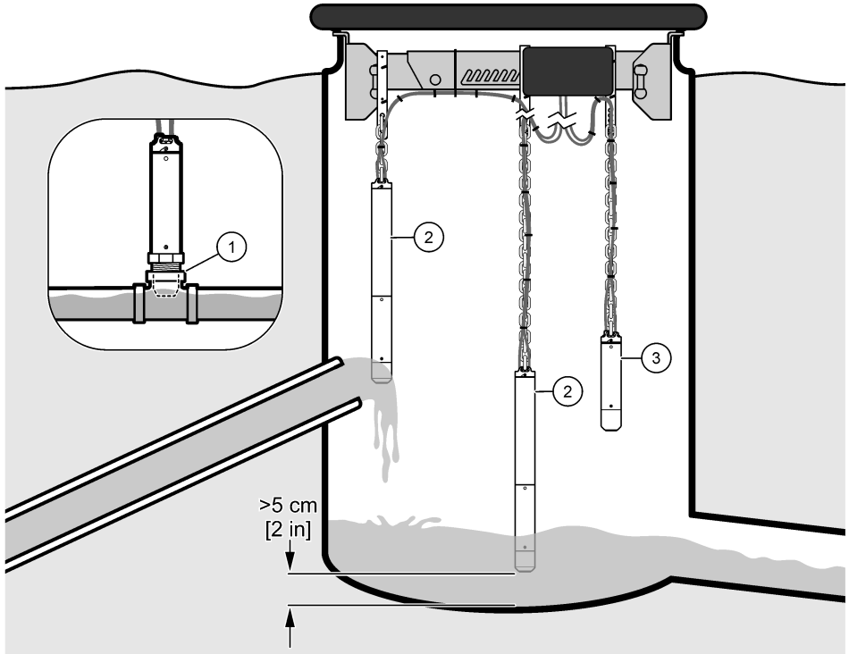
Abbildung 10 Inline oder frei hängend
