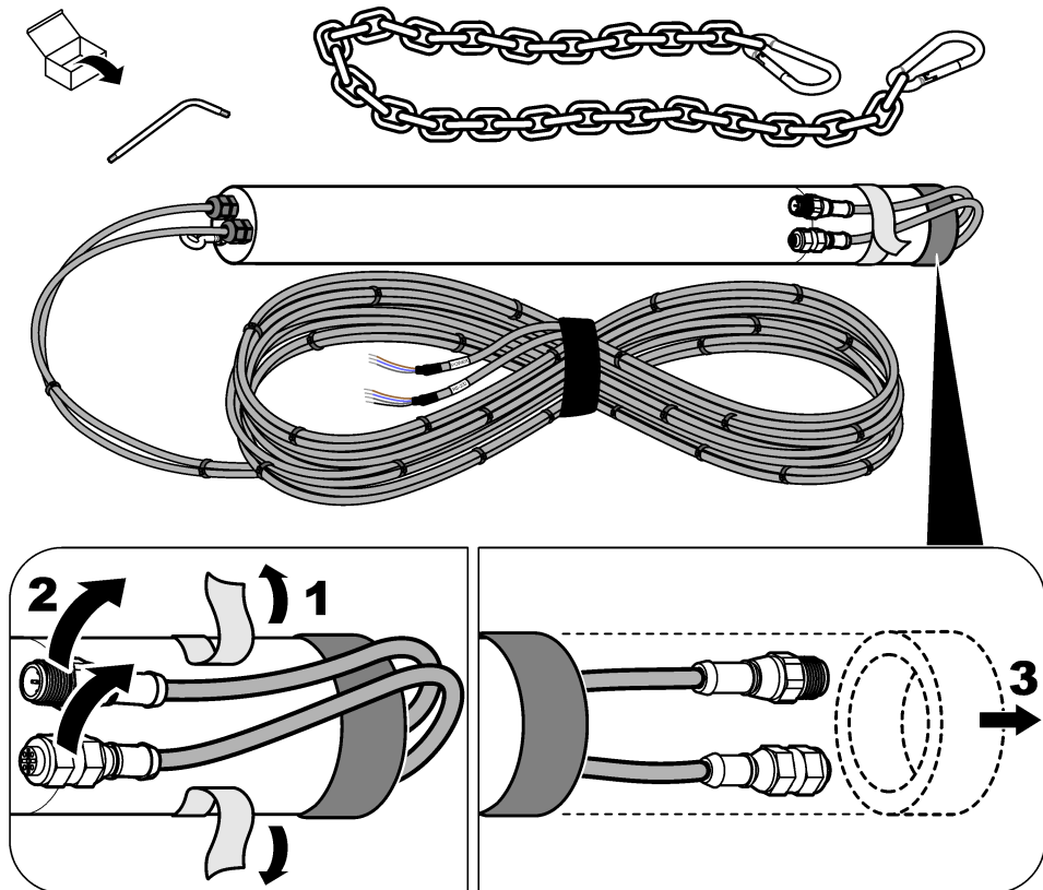
Figur 4 Feste kabelbeskytteren
