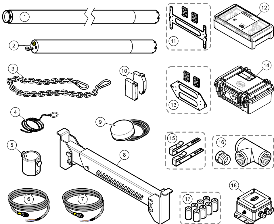
Obrázok 3 Príslušenstvo
