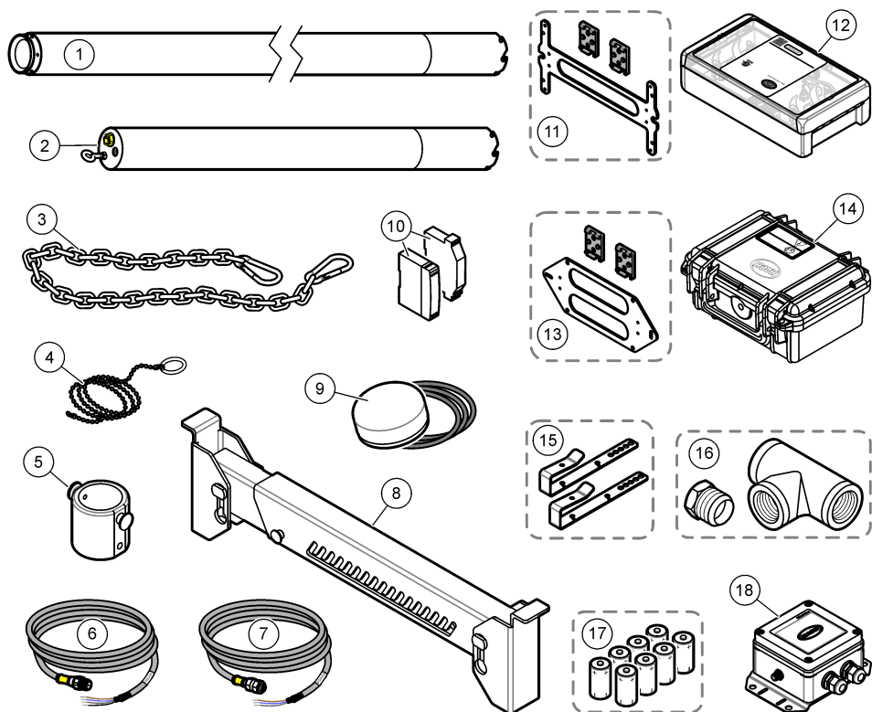
Obr. 3 Příslušenství
