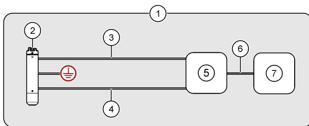
Slika 7 Prehod CDx440sc in kontrolna enota SC
