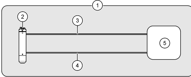
Şekil 8 Cihaz—Düz analog (4-20 mA) veya dijital (RS-232) iletişim
