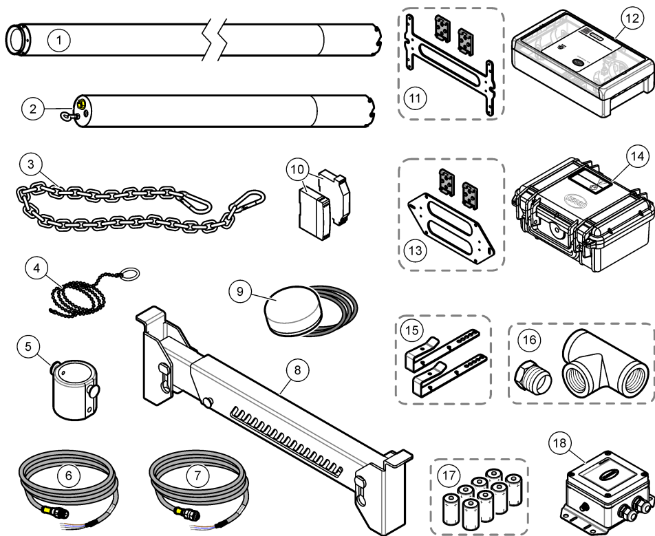
Figura 3 Accessori
